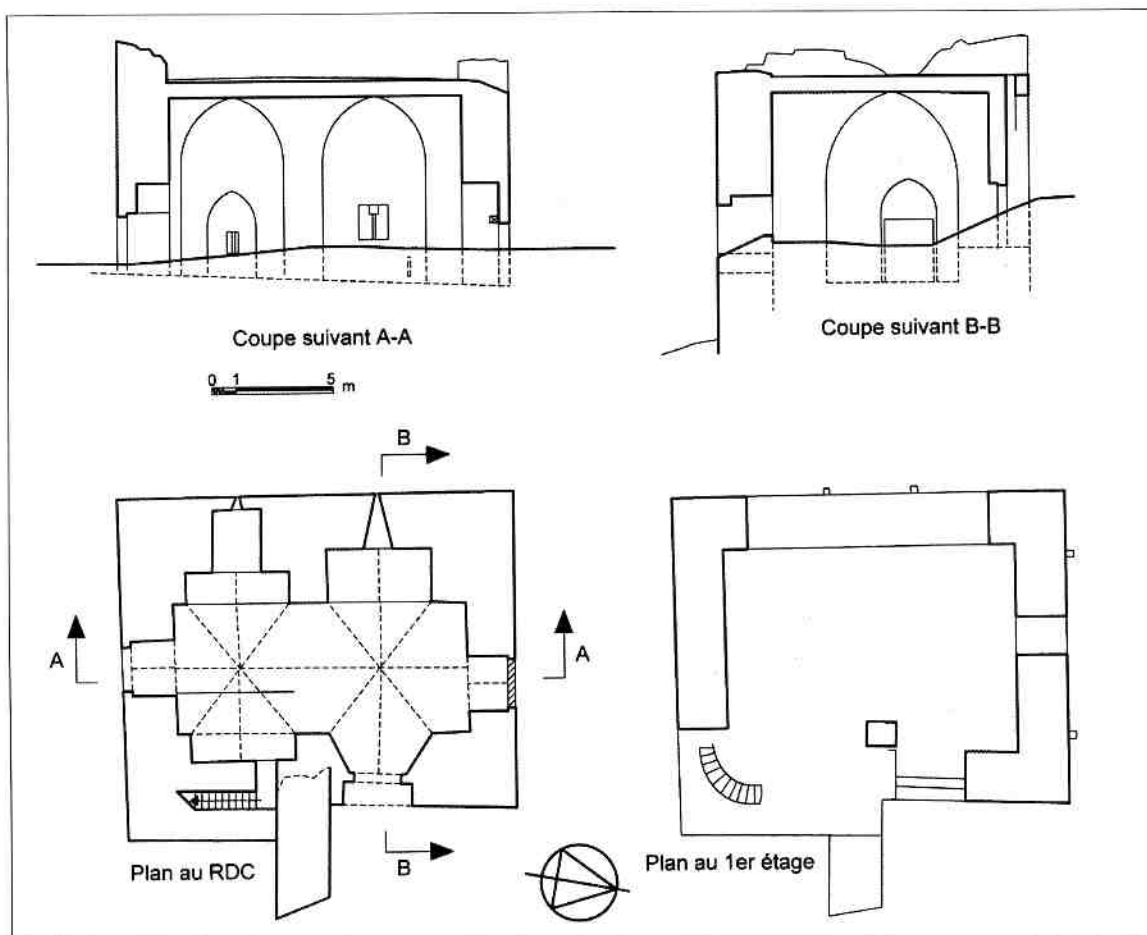
Plan 6 : Bourzey. Plans et coupes de la tour 3.
