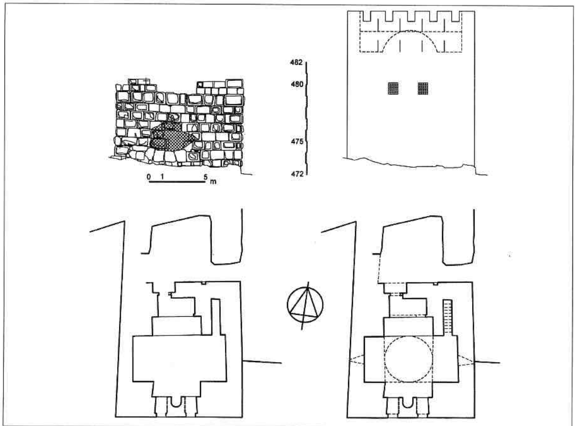
Plan 13 : Bourzey. Plans et élévations de la tour 20. Tour-mosquée. État actuel et restitution.
