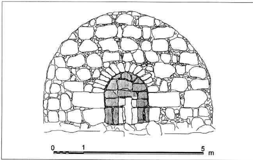
Plan 12 : Bourzey. Élévation de l'archère sud de la tour 8.
