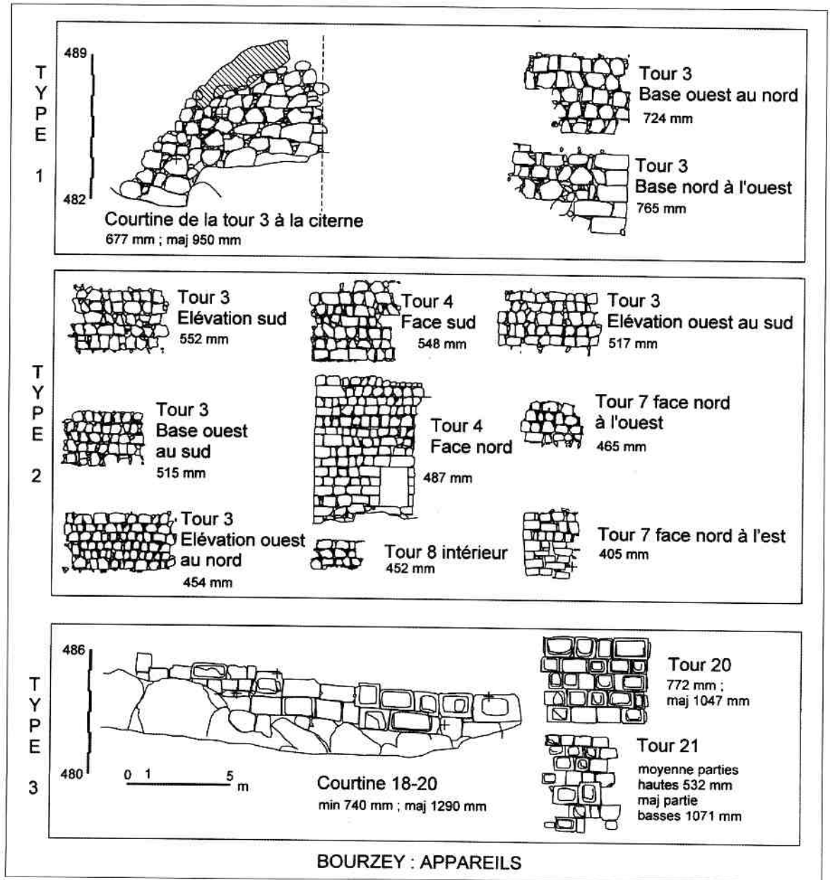
Plan 5 : Typologie des appareils de Bourzey.
