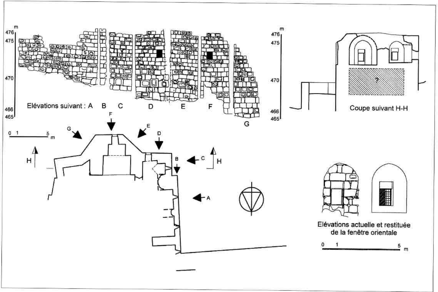
Plan 14 : Bourzey. Plan, élévations et coupes de la tour 21.
