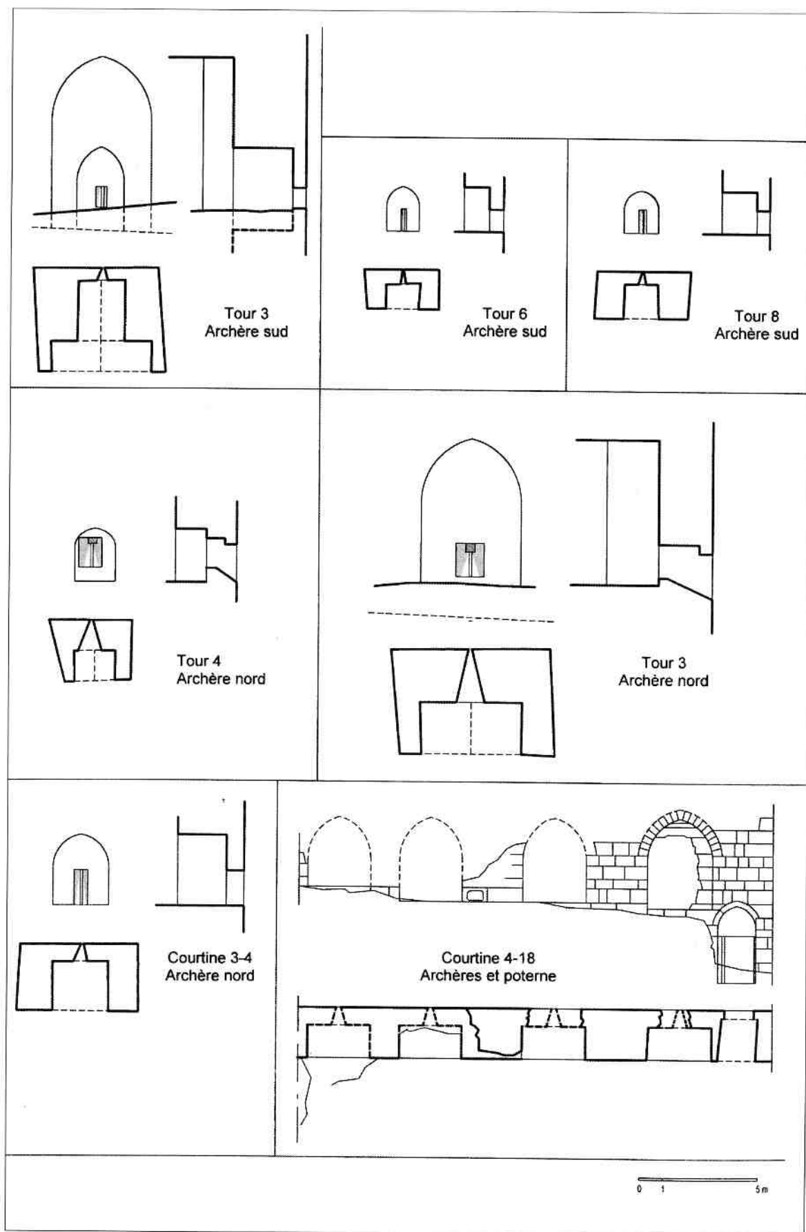
Plan 16 : Bourzey. Tableau synoptique des archères.
