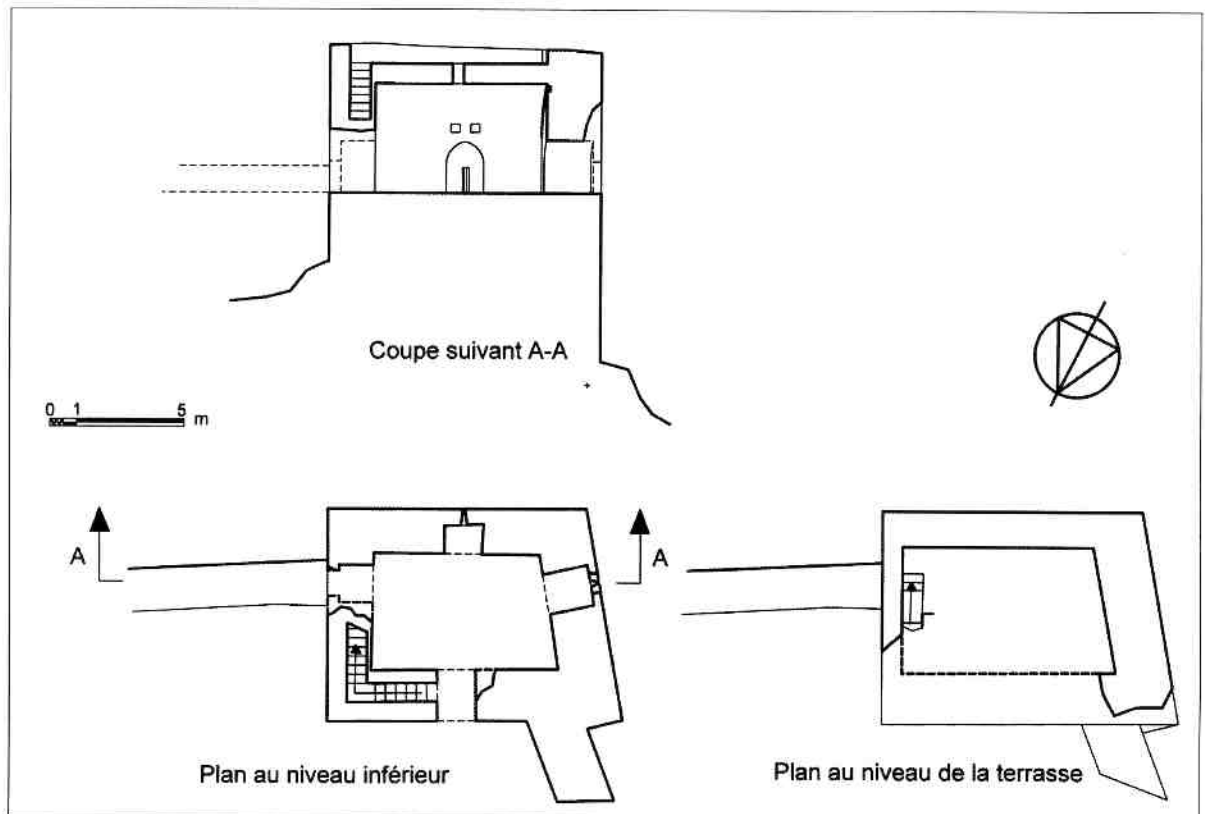
Plan 10 : Bourzey. Plans et coupe de la tour 6.
