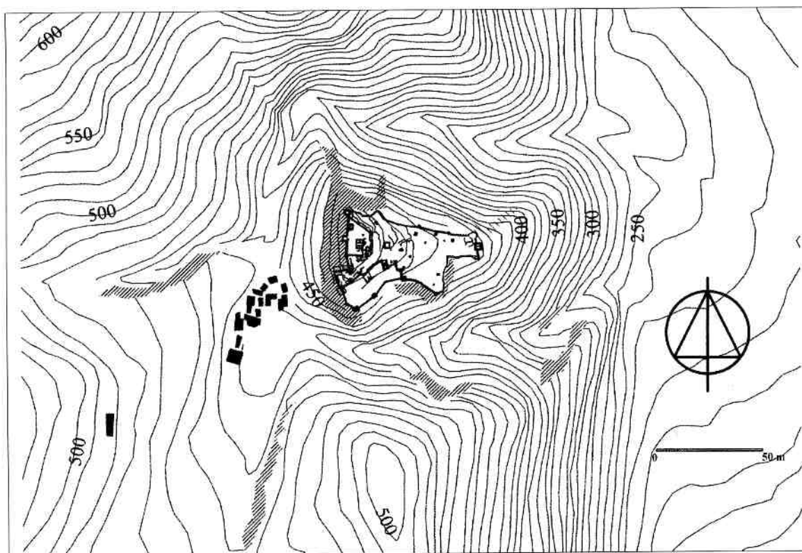
Plan 1 : plan général du site de Bourzey, d'après la carte d'état-major et les relevés de l'équipe.
