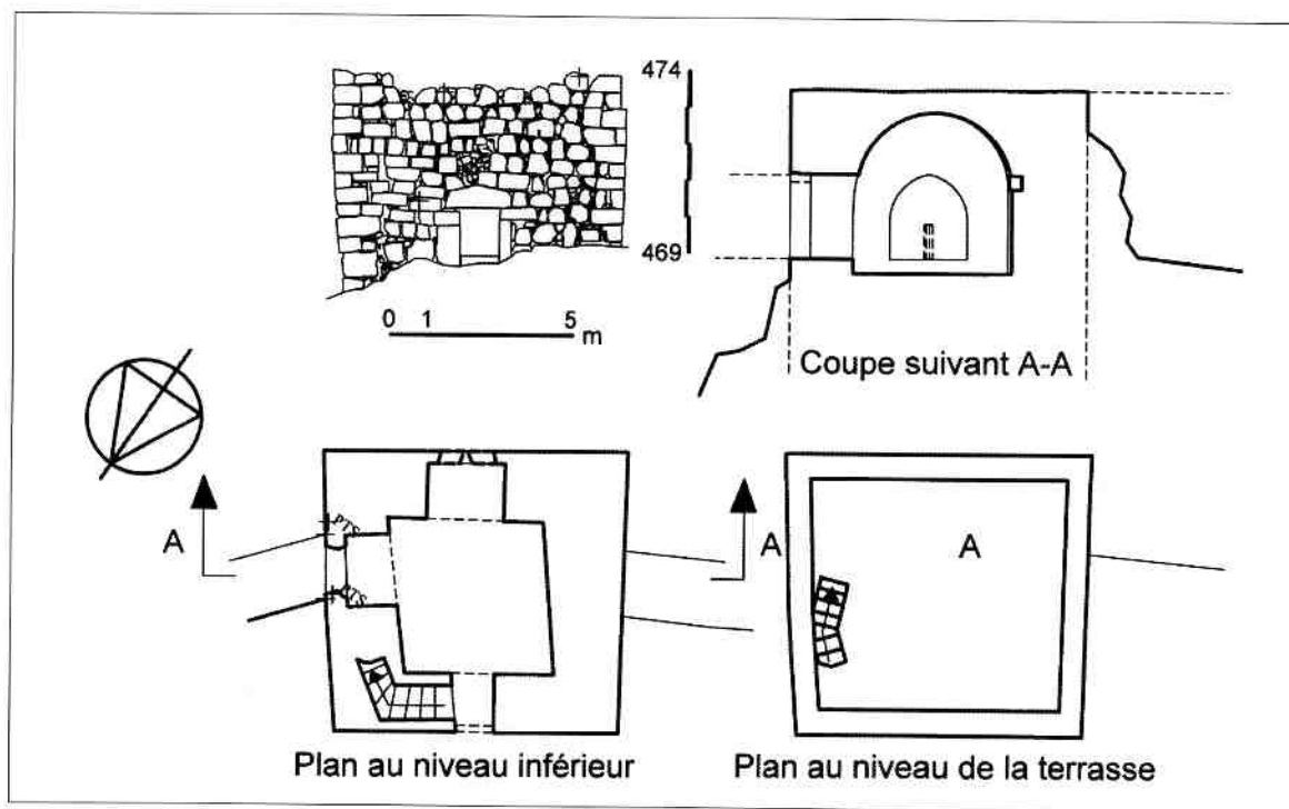
Plan 11: Bourzey. Plans, élévation et coupe de la tour 7.
