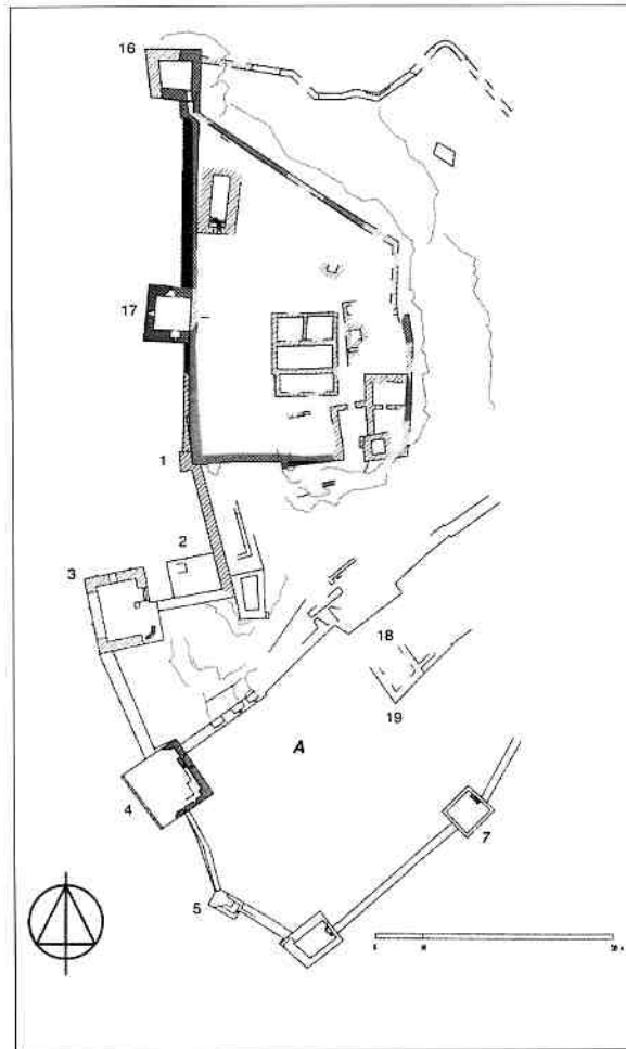
Plan 15 : Plan de la qulla. (Pour les couleurs par campagne, cf. cahier couleur, Mesqui plan 2).
